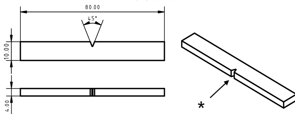
ISO 180 衝撃試験片 (単位 : mm)
