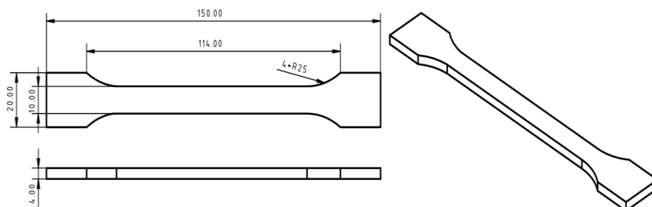
ISO 527 引張試験片 (単位 : mm)
